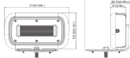
45W( Wall Mount)
